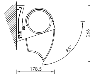
Montaggio a parete 85° Wall installation 85°
