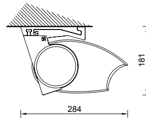
Montaggio a soffitto Ceiling installation
